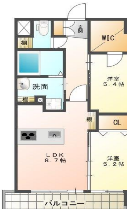
Iタイプ (50.6㎡)
